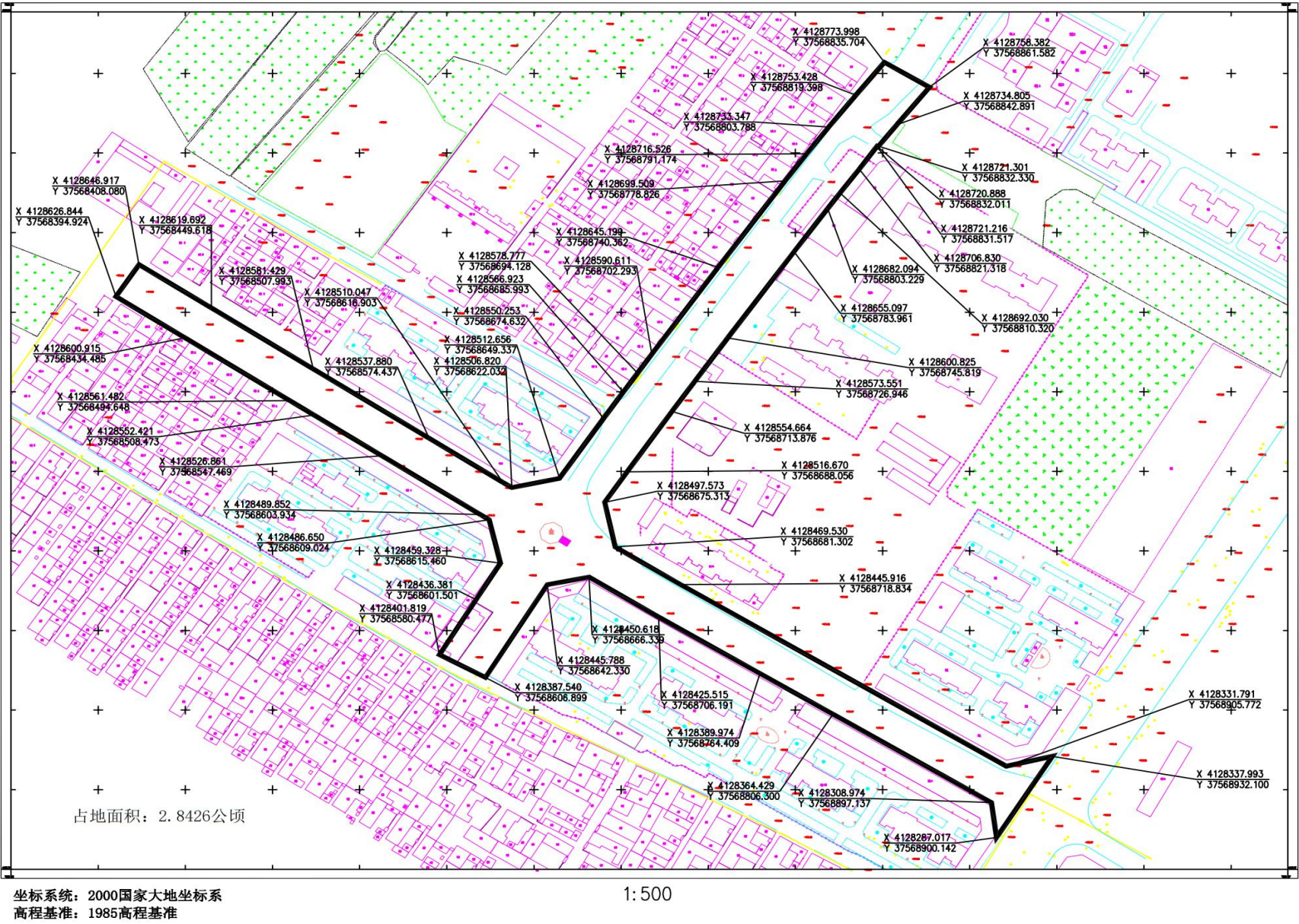
汾阳市冯家庄正街及西关路道路改造工程用地预审与选址平面图
